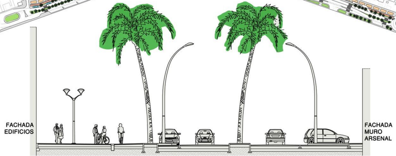
SECCION TIPO
