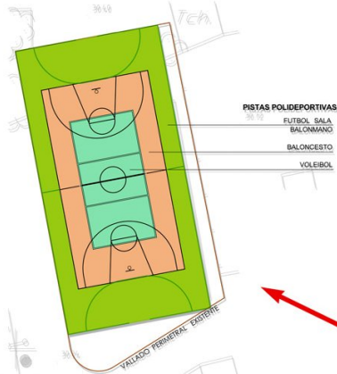
PROYECTO DE PISTA POLIDEPORTIVA EN LA APARECIDA PRESUPUESTO 37.455,43 € PLAZO DE EJECUCION 1 MES
