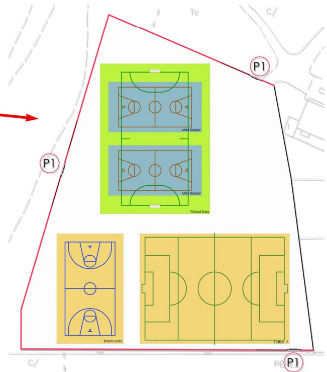
PROYECTO DE POLIDEPORTIVO BASICO EN LOS BELONES PRESUPUESTO 149.998,07 € PLAZO DE EJECUCION 3 MESES
