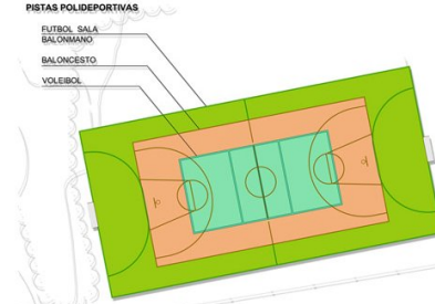
PROYECTO DE ACONDICIONAMIENTO DE ZONA DEPORTIVA EN PLAYA HONDA PRESUPUESTO 37.455,43 € PLAZO DE EJECUCION 1 MES
